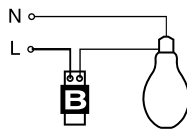
วงจรการต่อใช้งาน สำหรับหลอดไอปรอทความดันสูง
